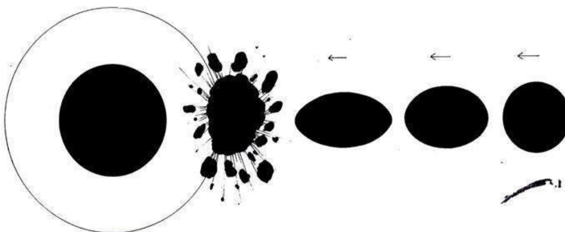
Fig.4. Roche limit
