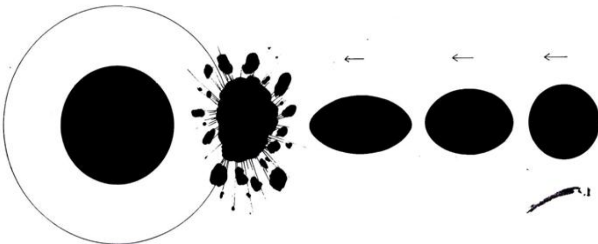
Fig. 4. Roche limit
